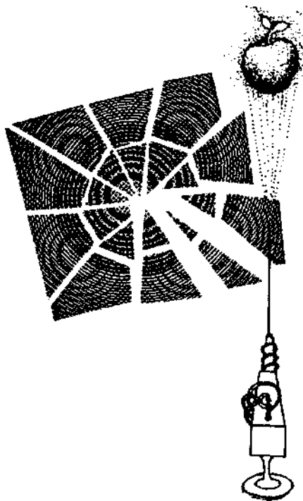
фиг. 4. За разлика от обикновената снимка, всяка част от холографската фотоплака съдържа цялата информация за цялото. Затова, ако една холографска плака се нахъса на парчета, всяко от тях може да бъде използвано за възстановяване на целия образ.
